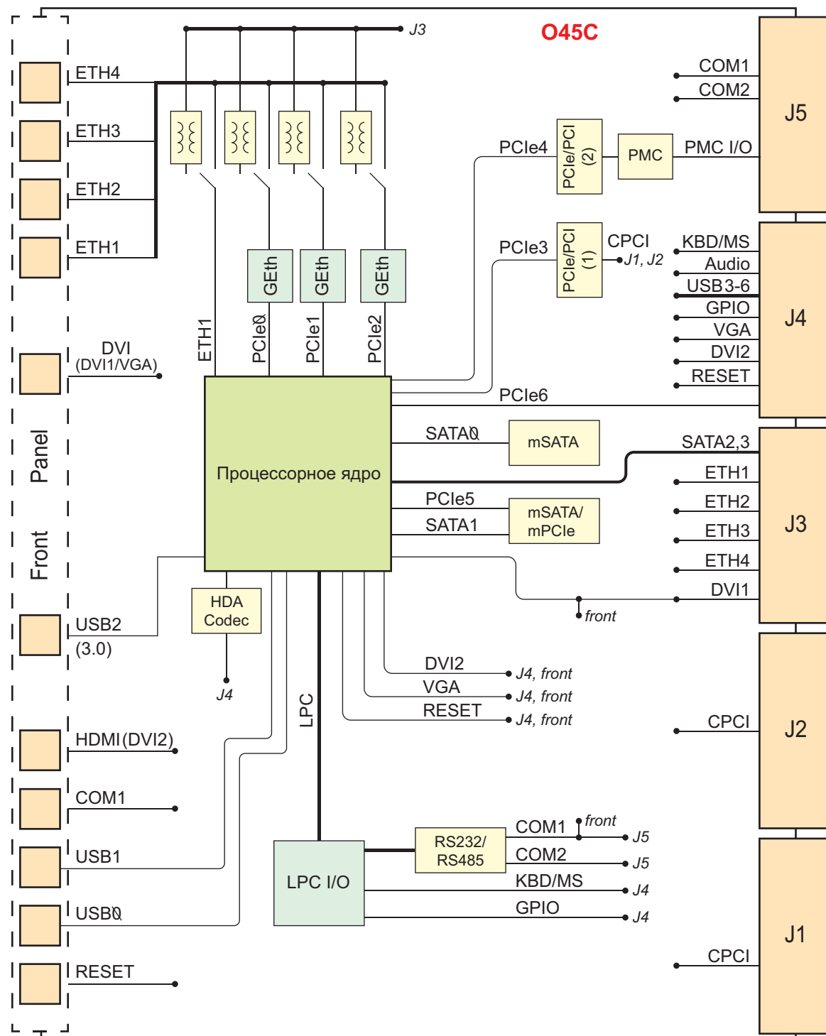
Структурная схема модуля О45С
