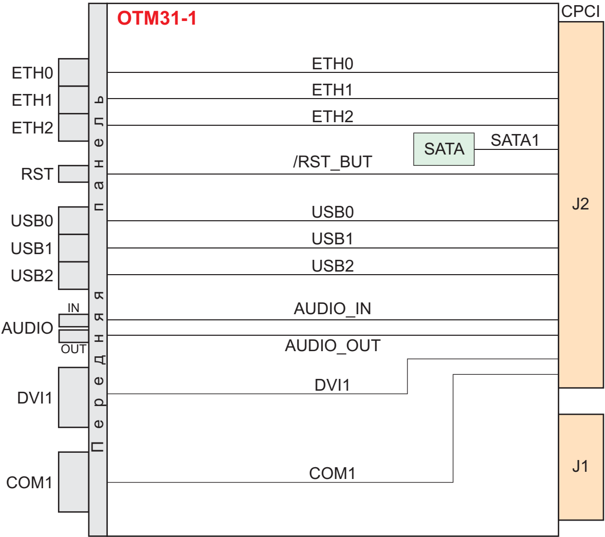
Структурная схема модуля OTM31C
